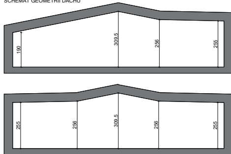
SCHEMAT GEOMETRII DACHU
